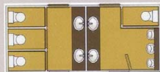
Plano distribución Maxilux.
